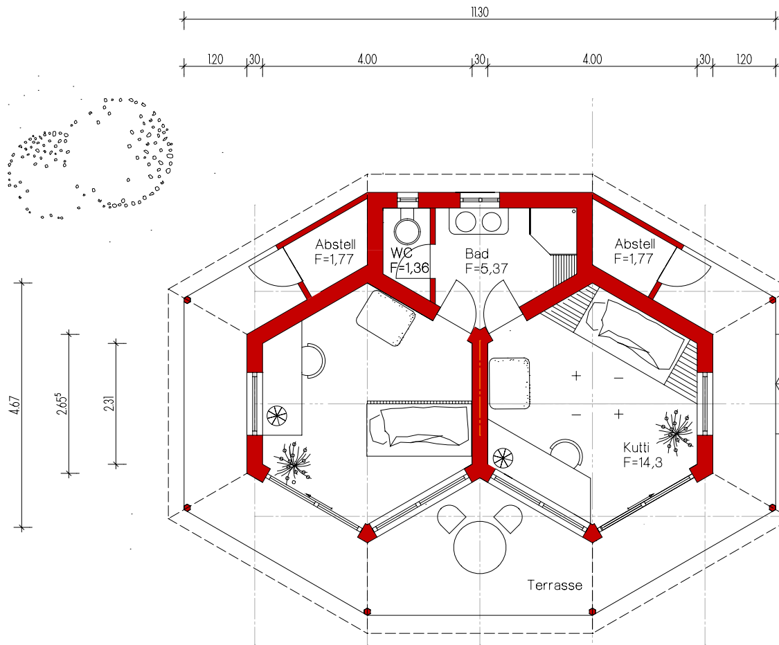
Grundriss Doppel-Kutti
